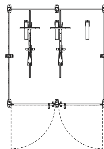
Module Be'Max 6 emplacements (L x P x h) : 2500 x 3000 x 2600 mm
