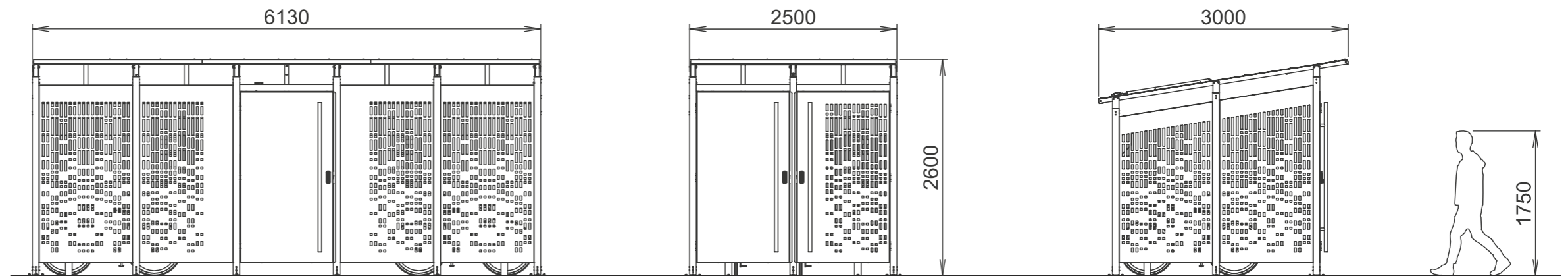
Module Be'Max 12 emplacements (L x P x h) : 6130 x 3000 x 2600 mm
