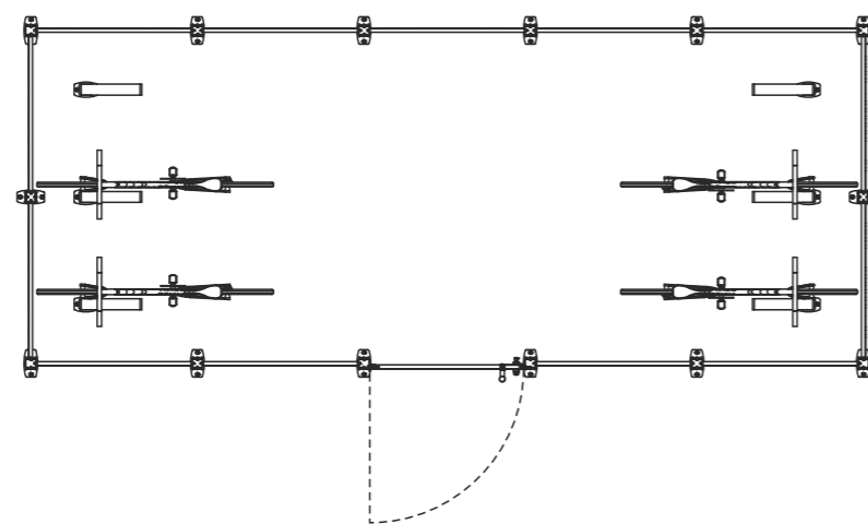
Module Be'Max 12 emplacements (L x P x h) : 6130 x 3000 x 2600 mm
